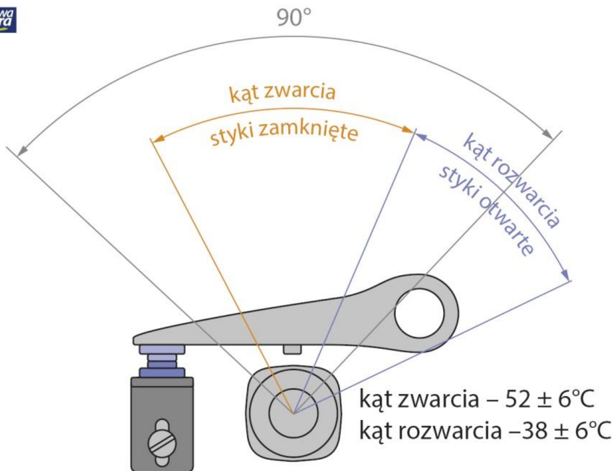
Ryc. 6.6. Graficzne przedstawienie kąta zwarcia i kąta rozwarcia styków
