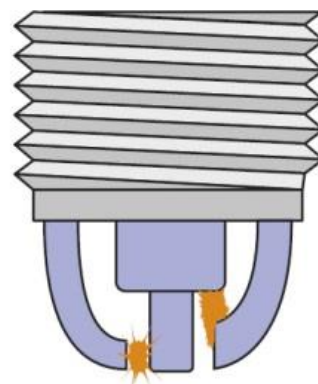
Ryc. 6.13. Rodzaje iskier w zależności od kształtu elektrody
